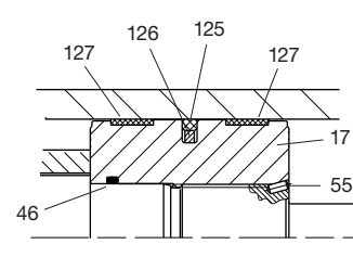
Standard-Kolben
