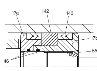
Dachmanschettenkolben
