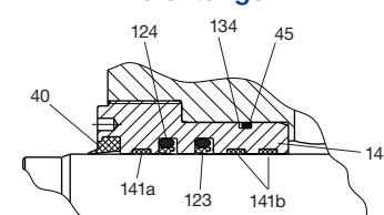
Reibungsarme Büchse und Dichtungen
