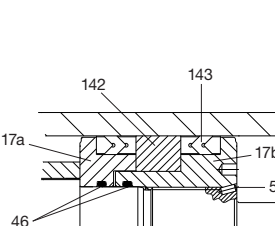
Dachmanschettenkolben
