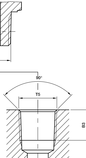
Einschraubloch BSPT (kegelig) ISO 7/1-Rc/BS 21-Rc DIN 2999-Rc (Japan: PT)
