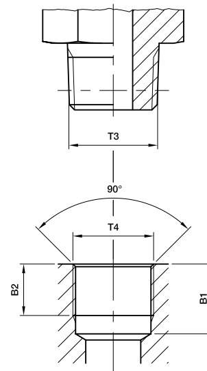
Einschraubloch (parallel) Metrisch DIN 3852-1 BSPP DIN 3852-2
